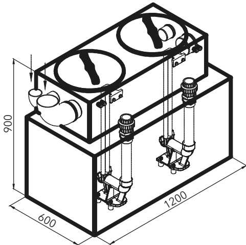
İKİLİ FOSEPTİK
