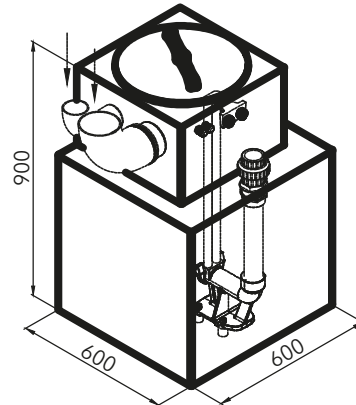
TEKLİ FOSEPTİK
