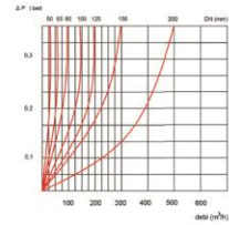
BASINÇ KAYBI GRAFİĞİ
